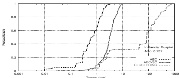
Figura 1: Análise empírica do AEC, AEC-SC, e CLUSTERING.
