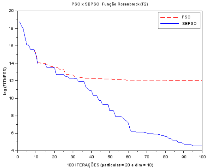
Figura 2. Na função f_2 , o PSO entra em estagnação perto da iteração 80, enquanto o SBPSO nas proximidades da iteração 95.
