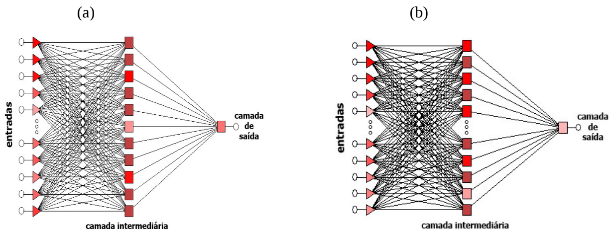
Figura 5: Arquiteturas das redes otimizadas com as seguintes estruturas neurais 19-11-1 para (a) Cananéia e 22-11-1 para (b) Ponta da Armação [11].
