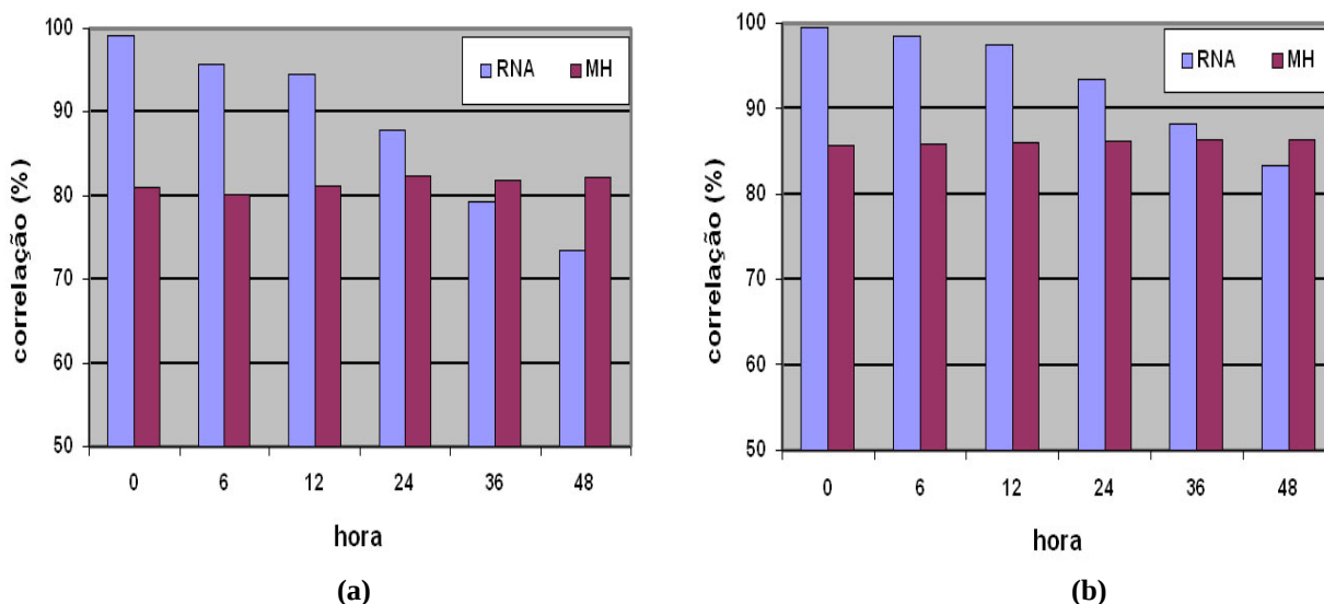
Figura 8: Correlações entre a RNA e o MH para previsões até 48 horas (a) para Cananéia e (b) para Ponta da Armação [11].
