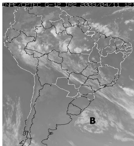
Figura 2: Imagem de satélite do dia 11 de abril de 2003 (09:00 HL) - INPE/CPTEC.
