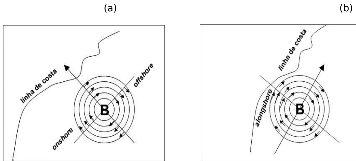
Figura 1: (a) Circulação ciclônica deslocando-se em direção perpendicular à costa (Furacão). (b) Circulação ciclônica deslocando-se paralela à costa (ciclones extratropicais), sendo o tipo de tormenta mais freqüente no HS [11].
