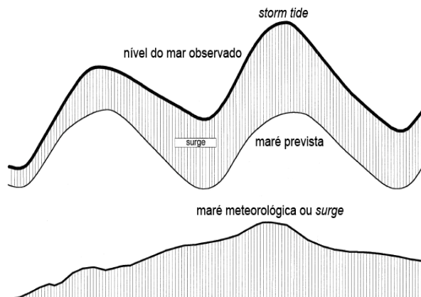
Figura 3: Curvas referentes às variações nas alturas do nível do mar devidas às forçantes meteorológicas e astronômicas, verificadas a partir dos registros maregráficos, adaptado de [2].
